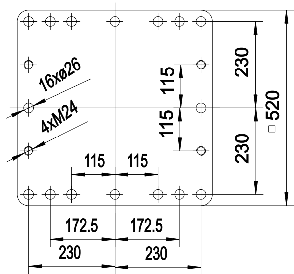
Kiinnitysmitat Fastening dimensions 1:10
