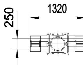
Kiinnitysmitat Fastening dimensions 1:10
