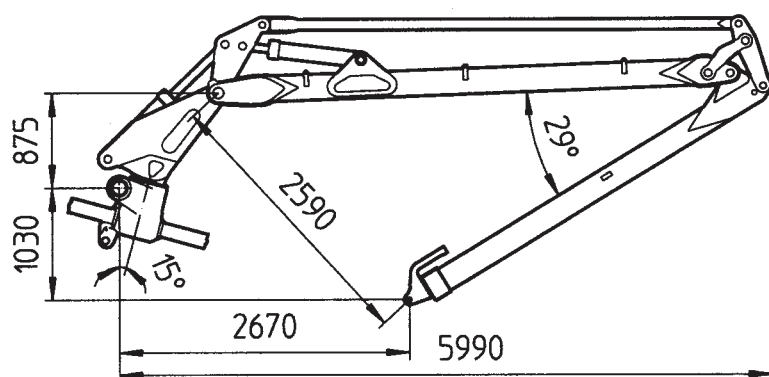
Kuljetusasento, Transport position
