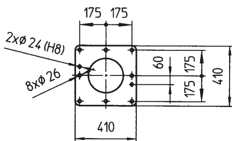
Kiinnitysmittat Fastening dimensions
